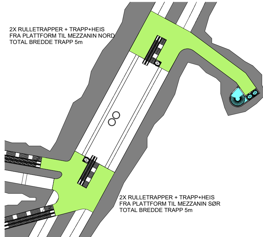
Nivå Mezzanin 1 : 500
