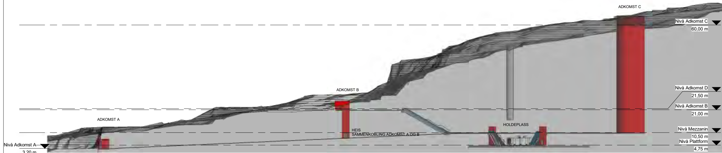
Snitt Holdeplass og Adkomst 1 : 500
