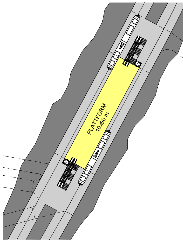
Nivå Plattform 1 : 500
