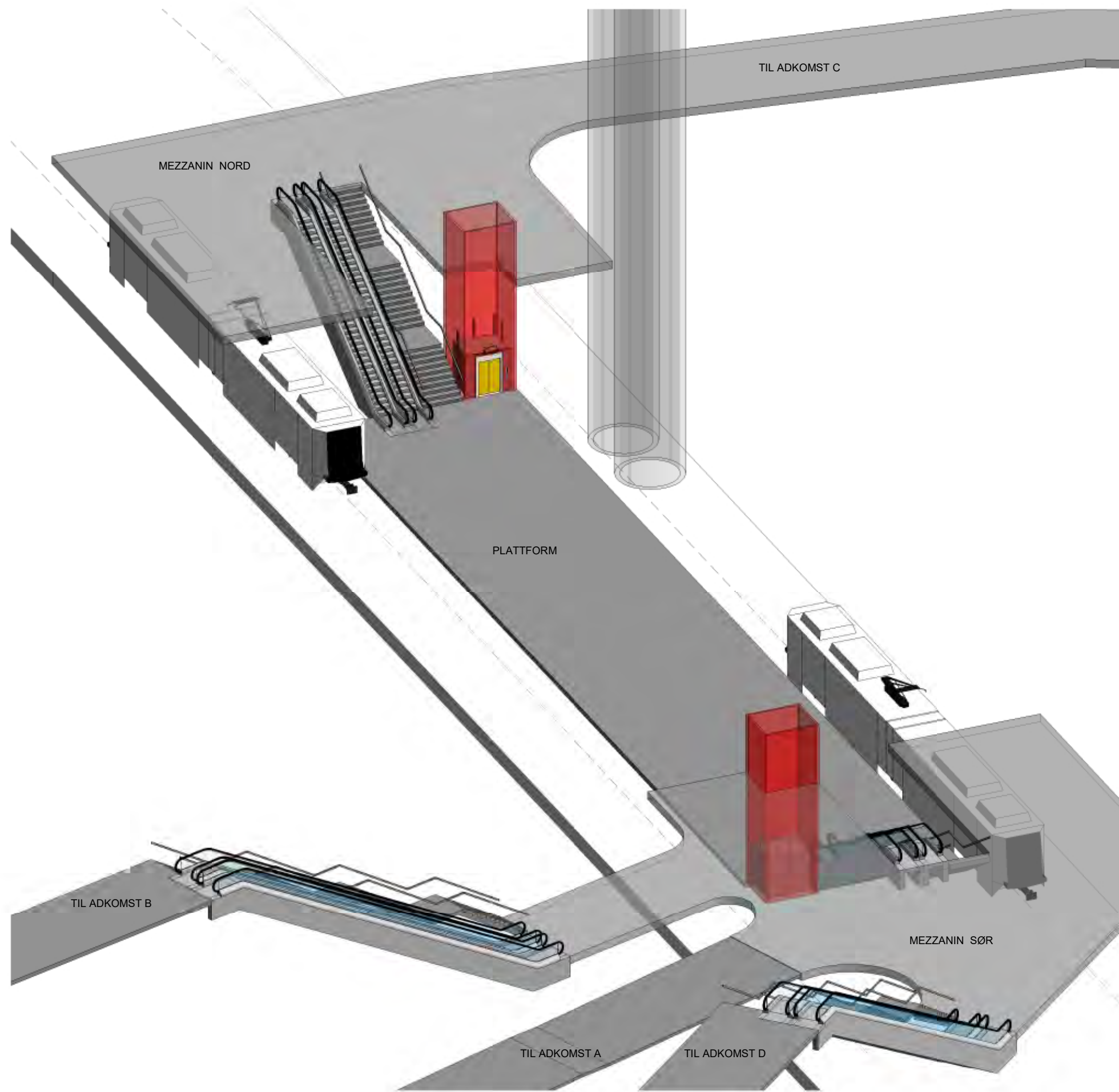
3D Illustrasjon Holdeplass
