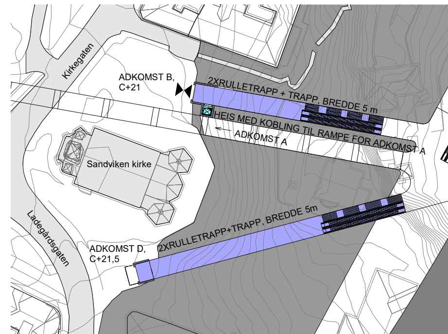
Adkomst B og D 1 : 500
